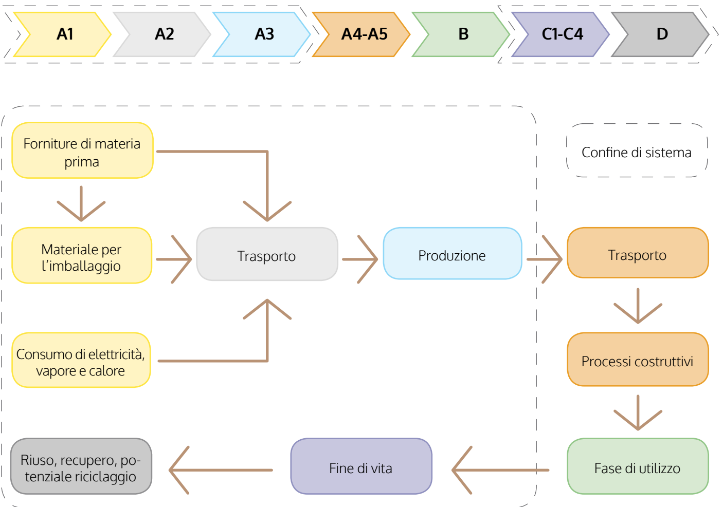
Figura 1 Limite di sistema dello studio LCA condotto su BetonWood® , pannello in cementolegno
